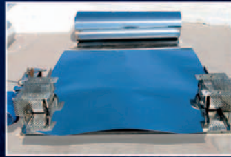
Profilieren der Edelstahlbänder.
